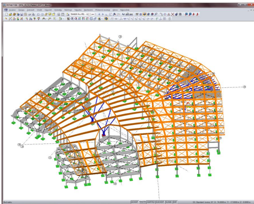
Část konstrukce navrhovaná v programu RSTAB.
